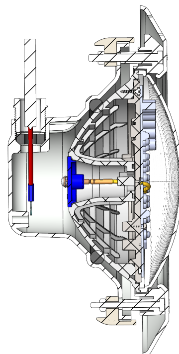
SECCIÓN A-A
